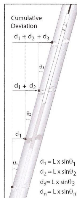
Fig. 3: rappresentazione schematica dello spostamento misurato ad ogni stop di misura. Fig. 4: rappresentazione schematica dello spostamento cumulativo misurato in un tratto di TIV
